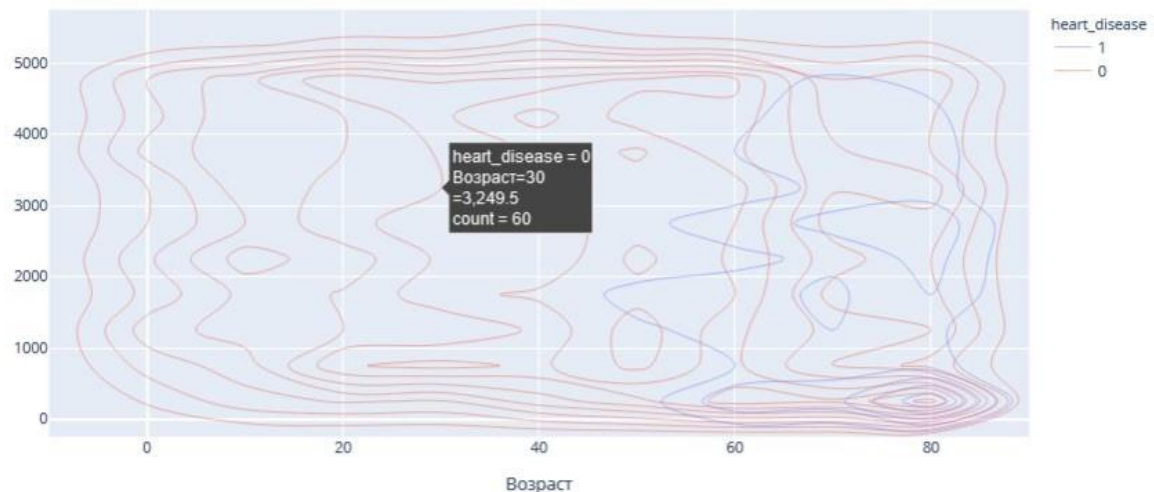
График возрастов пациентов на основе сердечных заболеваний
